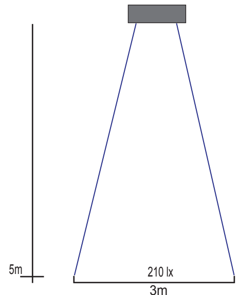
Rozkład nateżenia oświetlenia / -Distance Curve
