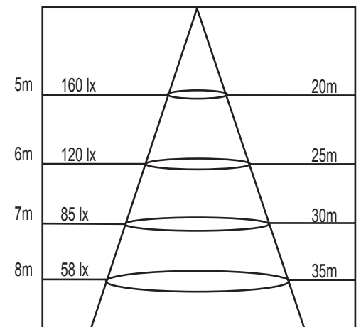
Rozkład nateżenia oświetlenia / -Distance Curve
